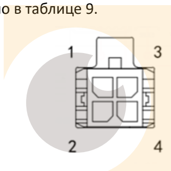
Рисунок 8 – Разъем подключения динамика/микрофона TTS
