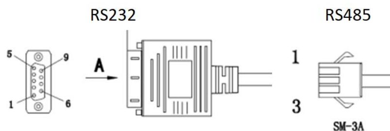
Рисунок 7 – Разъем I/O2
