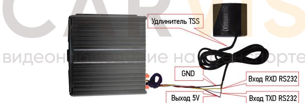
Рисунок 19 – Подключение TTS (Text To Speech)
