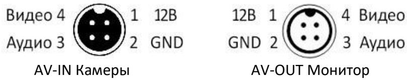
Рисунок 5 – Разъемы подключения камер и монитора
