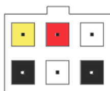
Рисунок 3 – Разъем кабеля питания
