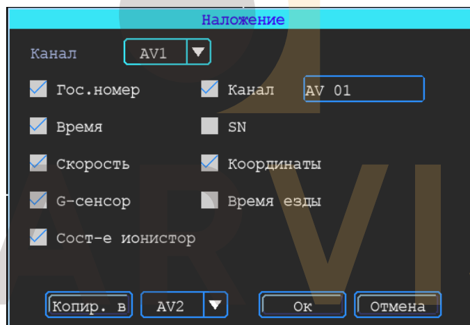
Рисунок 51 – Вкладка «Наложение»
