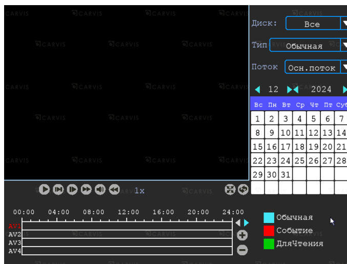
Рисунок 23 – Вкладка «Видео»
