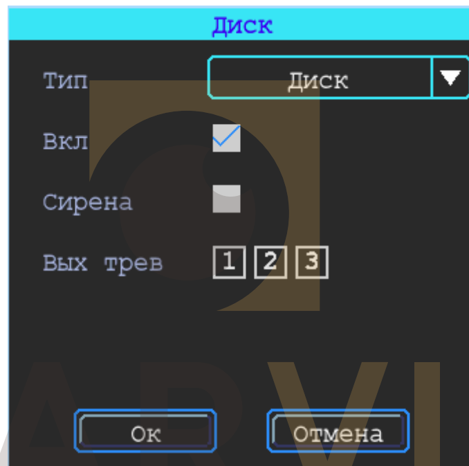
Рисунок 78 – Вкладка «Диск»
