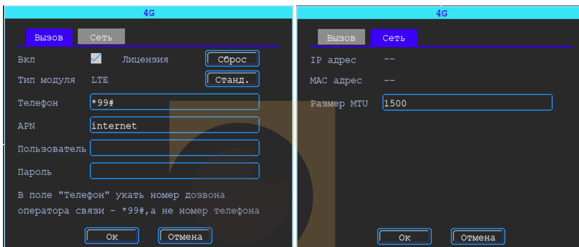
Рисунок 37 – Вкладка «3G/4G»
