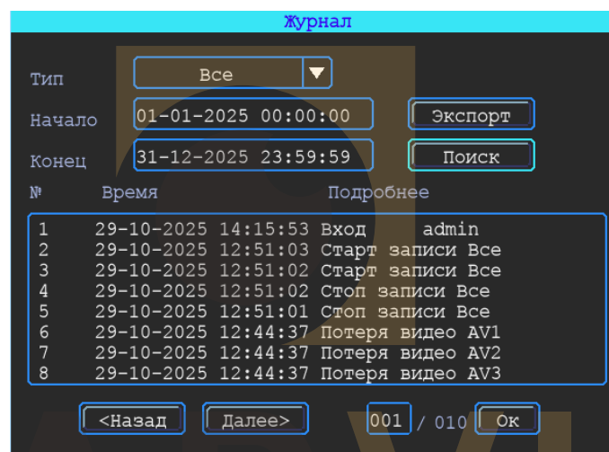
Рисунок 65 – Вкладка «Журнал»
