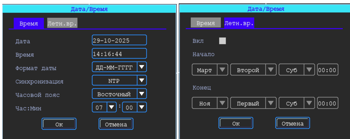
Рисунок 28 – Вкладка «Дата/Время»
