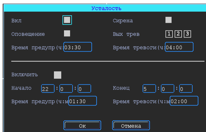
Рисунок 76 – Вкладка «Усталость»
