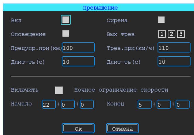
Рисунок 77 – Вкладка «Превышение»
