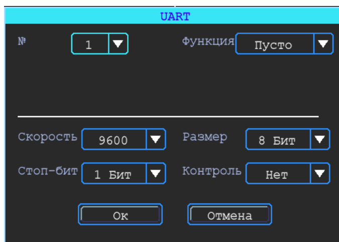
Рисунок 60 – Вкладка «UART»
