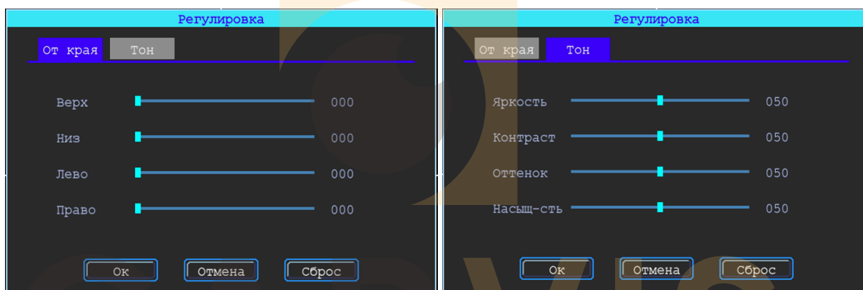
Рисунок 31 – Вкладка «Регулировка»
