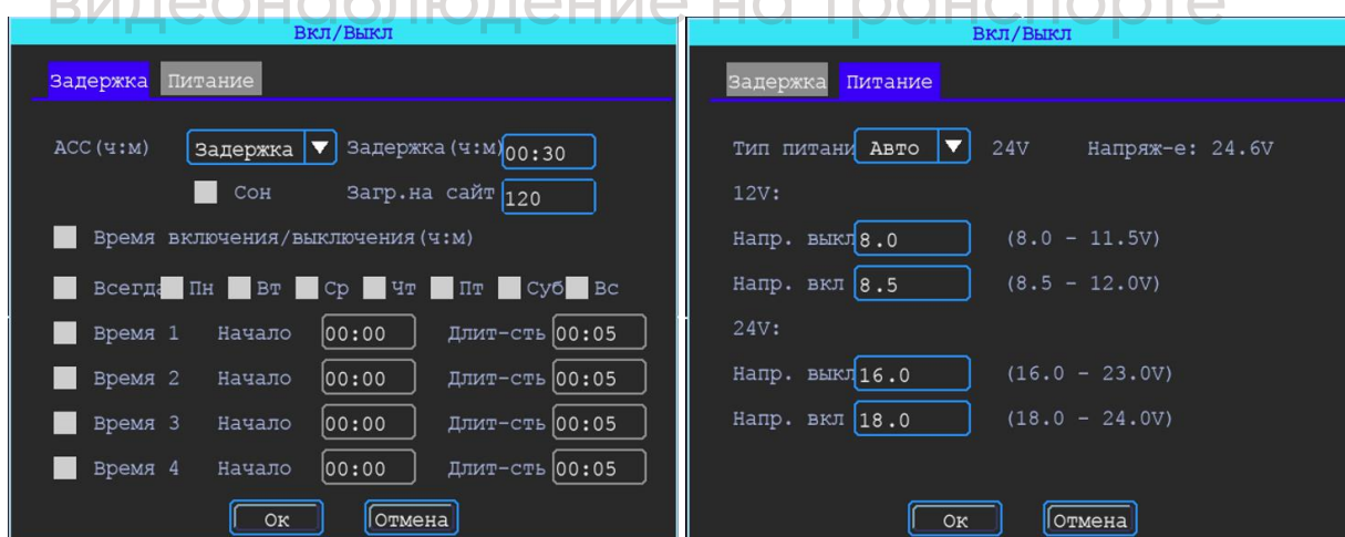
Рисунок 32 – Вкладка «Вкл/Выкл»
