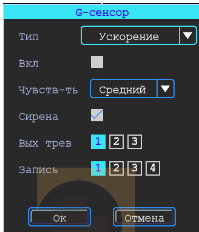
Рисунок 81 – Вкладка «G-сенсор»
