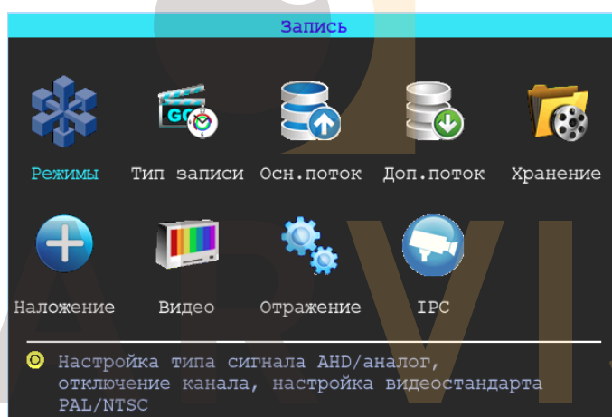
Рисунок 43 – Окно «Запись»
