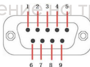
Рисунок 7 – Разъём интерфейса RS-232
