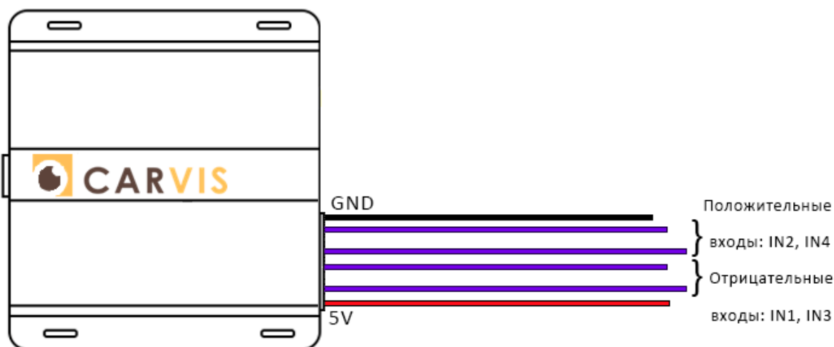
Рисунок 13 – Тревожные входы регистратора
