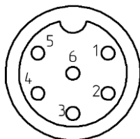
Рисунок 6 – Разъём подключения IP-камер и сети LAN
