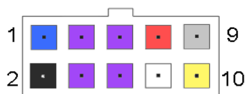
Рисунок 4 – Интерфейсный разъем
