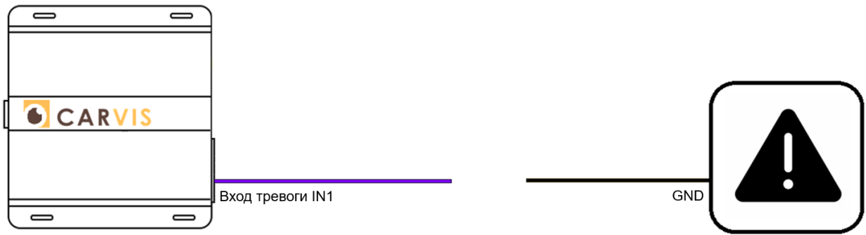
Рисунок 16 – Подключение тревожной кнопки
