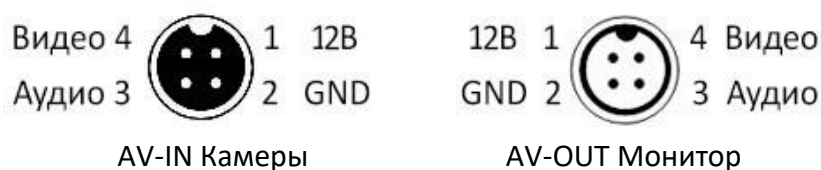
Рисунок 5 – Разъёмы подключения камер и монитора
