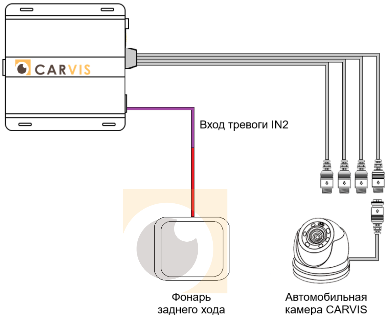
Рисунок 14 – Подключение тревожного входа к питанию фар заднего хода
