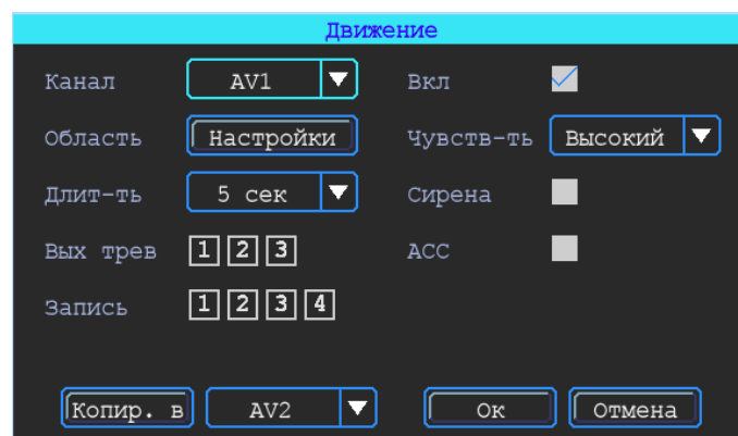
Рисунок 79 – Вкладка «Движение»
