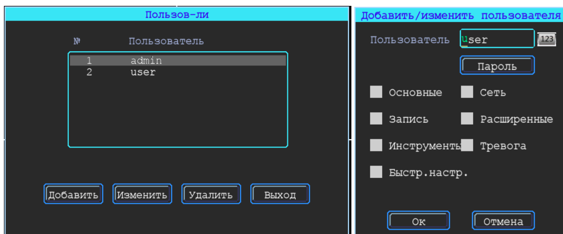
Рисунок 58 – Вкладка «Пользователь»
