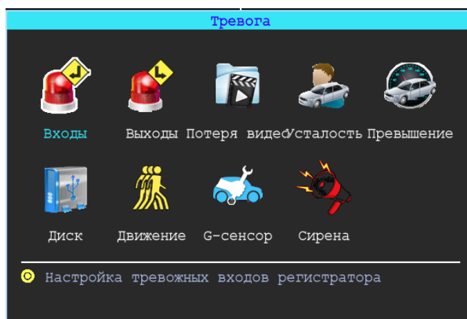
Рисунок 70 – Окно «Тревога»
