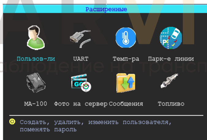
Рисунок 57 – Окно «Расширенные»
