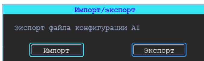
Рисунок 88 – Вкладка «Импорт/Экспорт»
