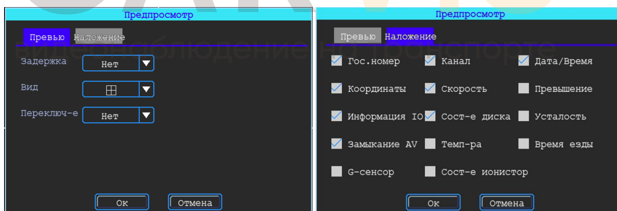
Рисунок 30 – Вкладка «Предпросмотр»
