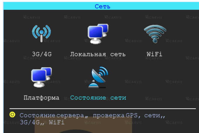
Рисунок 35 – Окно «Сеть»
