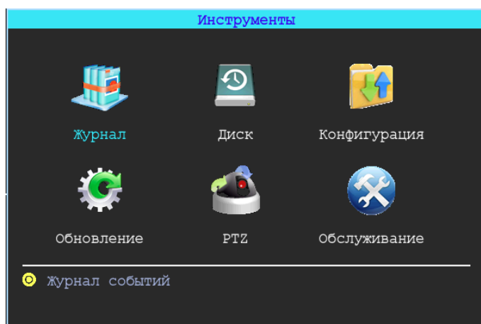
Рисунок 64 – Окно «Инструменты»
