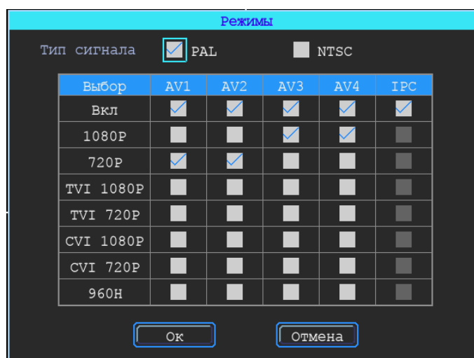
Рисунок 44 – Вкладка «Режимы»
