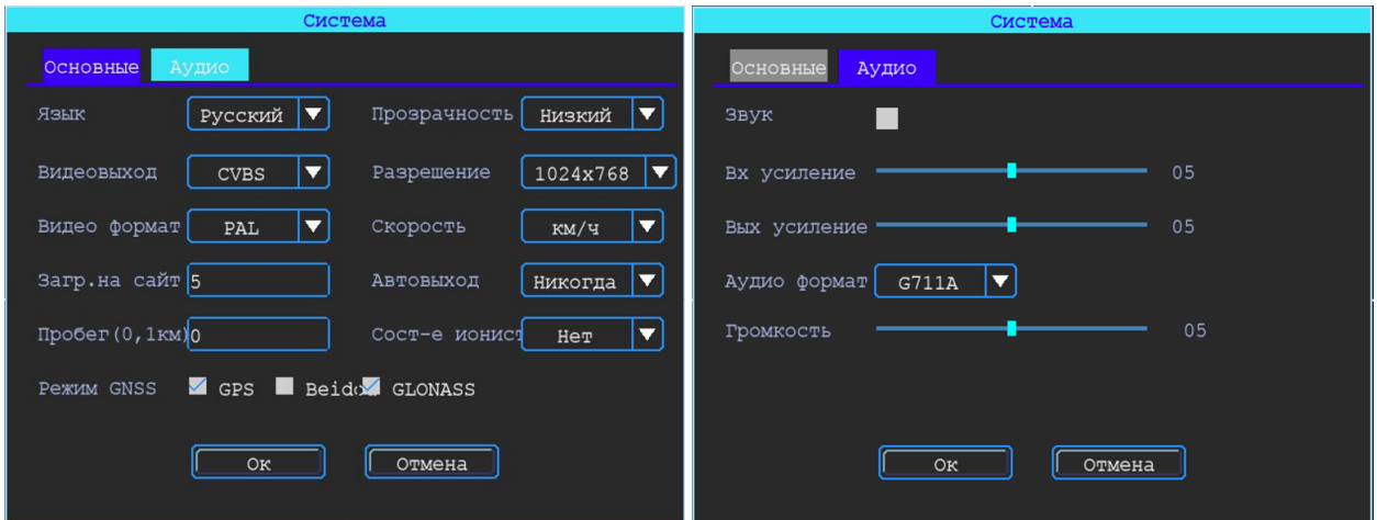
Рисунок 33 – Вкладка «Система»
