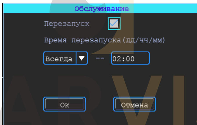
Рисунок 69 – Вкладка «Обслуживание»
