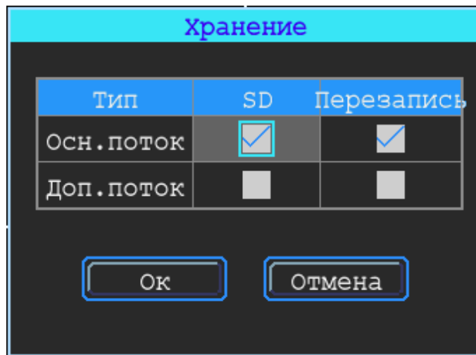
Рисунок 50 – Вкладка «Хранение»
