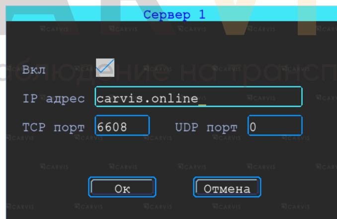
Рисунок 36 – Вкладка «Сервер»
