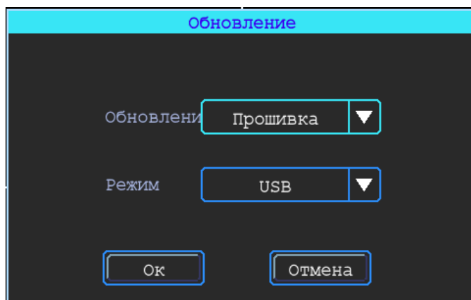
Рисунок 68 – Вкладка «Обновление»
