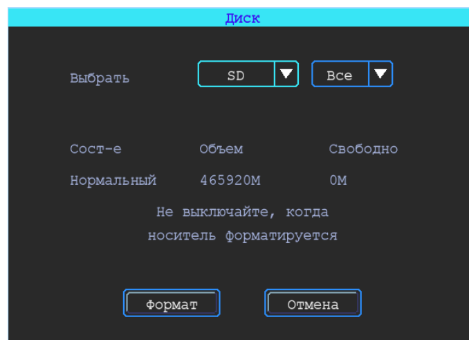
Рисунок 66 – Вкладка «Диск»
