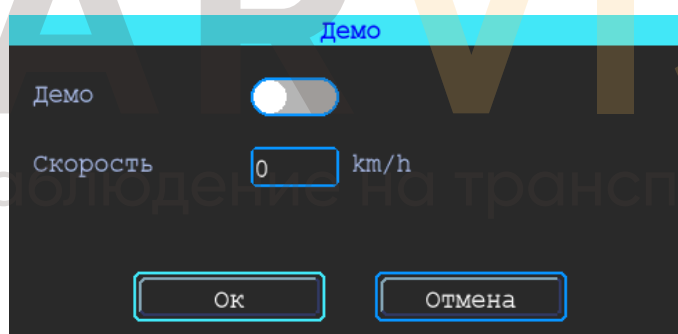
Рисунок 87 – Вкладка «Демо»
