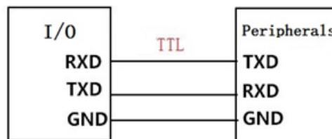
Рисунок 18 – Схема подключения последовательного порта
