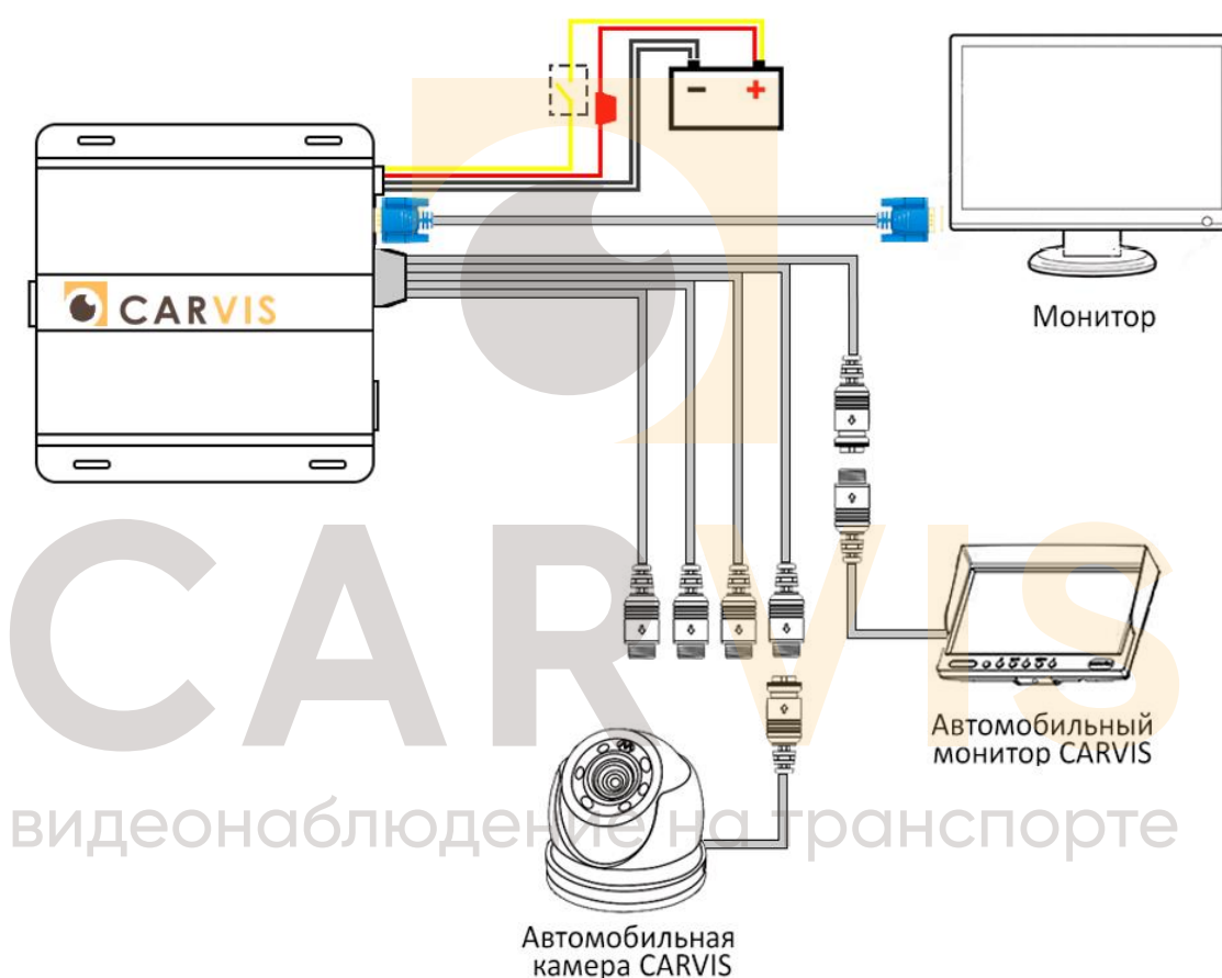
Рисунок 12 – Подключение питания
