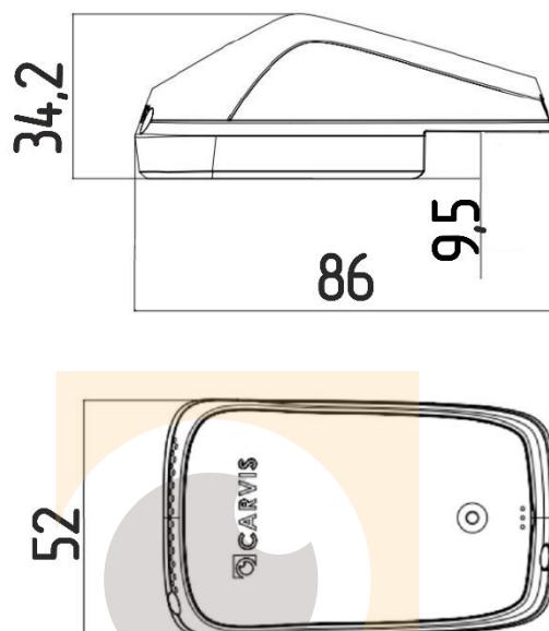
Рисунок 1 – Габаритные размеры и внешний вид камеры CARVIS MC-4213
